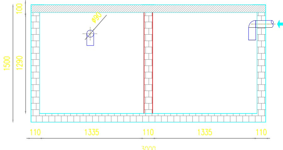
MẶT CẮT D-D
