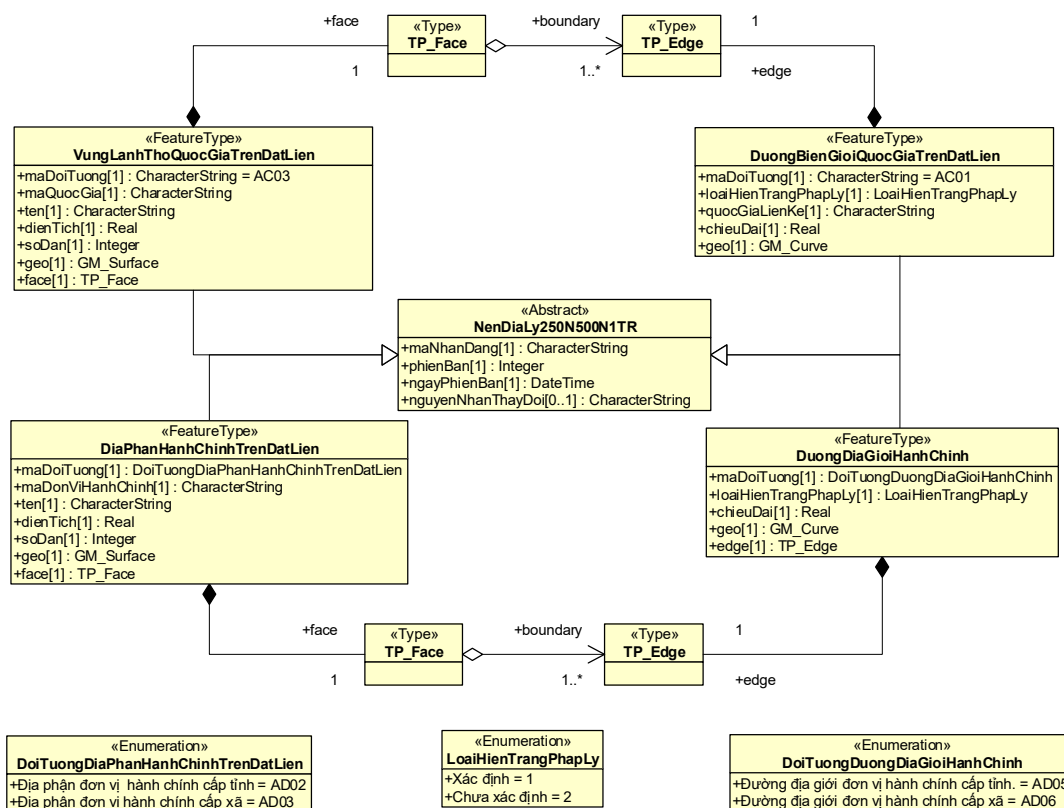
Hình 4. Lược đồ ứng dụng mô tả các lớp đối tượng địa lý trong gói dữ liệu biên giới, địa giới 3
