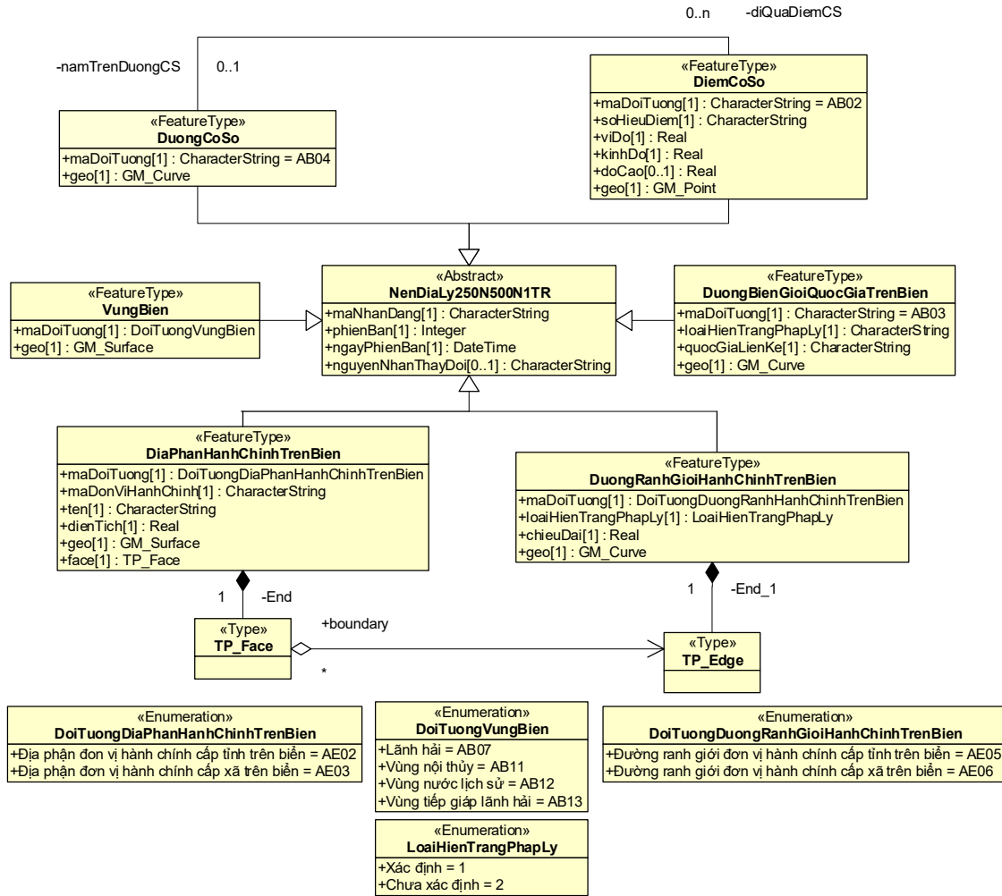
Hình 4. Lược đồ ứng dụng mô tả các lớp đối tượng địa lý trong gói dữ liệu biên giới, địa giới (kết thúc) 4
