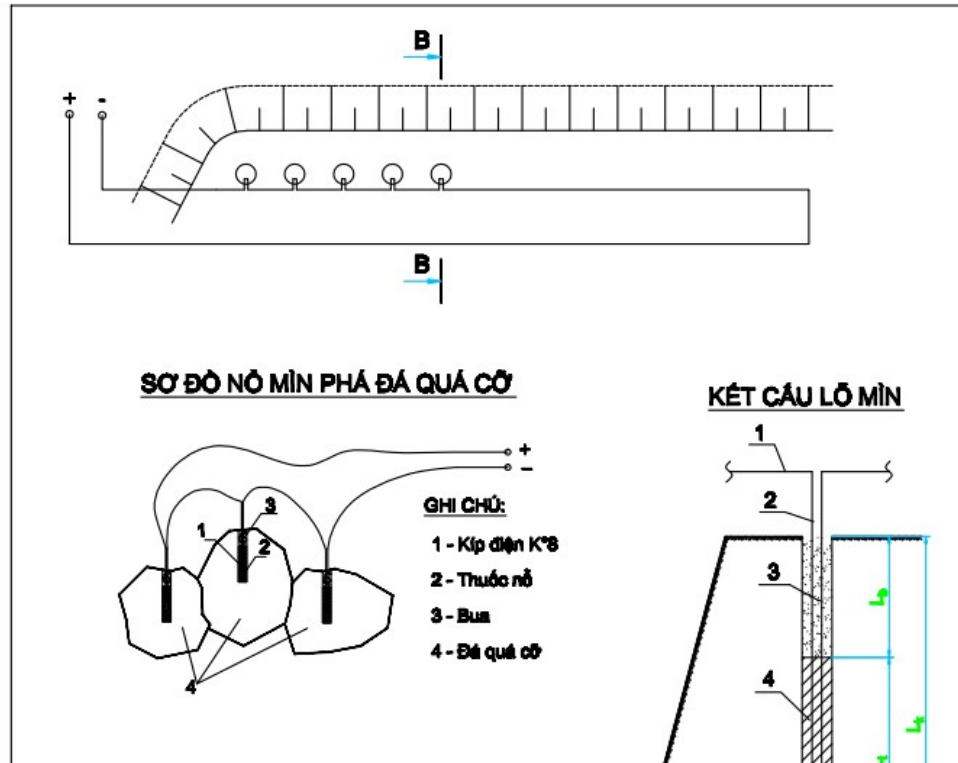
Hình 1. 6. Sơ đồ khoan nổ mìn
