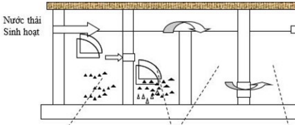
Hình 3. 1. Sơ đồ bể tự hoại
