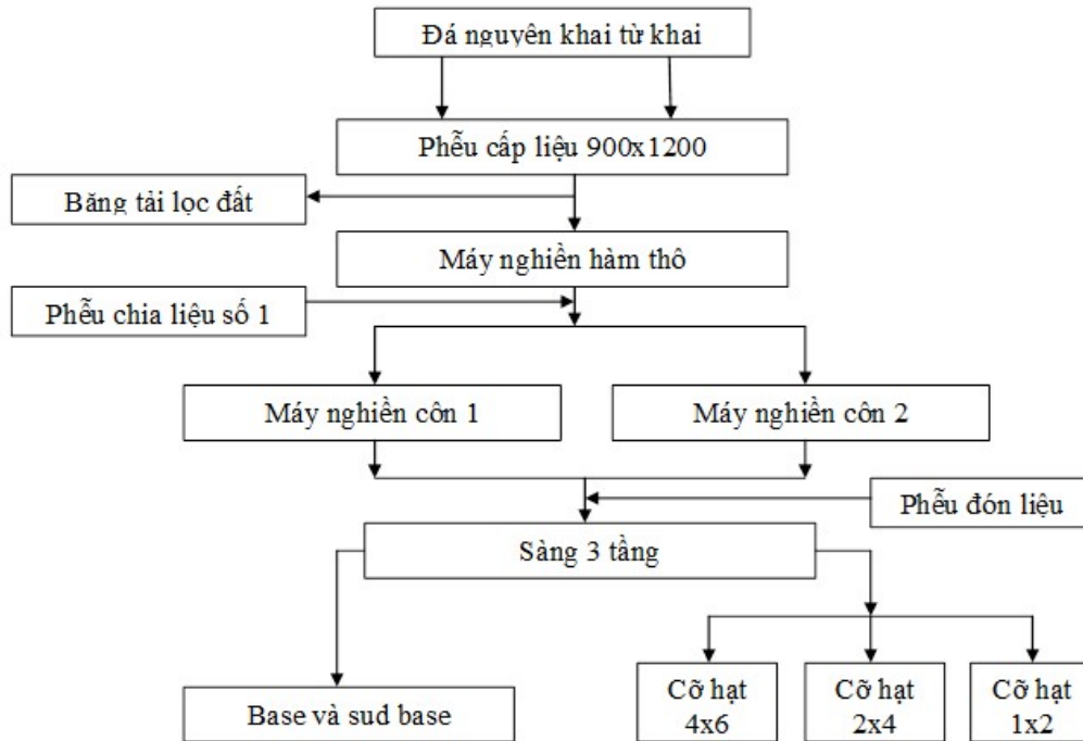
Hình 1. 7. Sơ đồ chế biến đá Dự án khai thác đá
