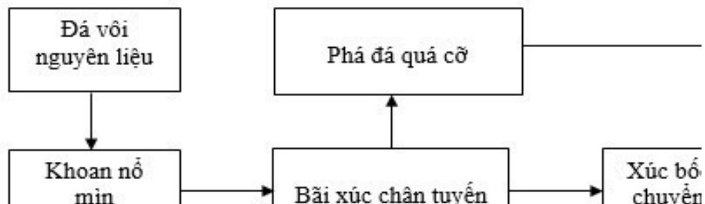
Hình 1.3. Sơ đồ công nghệ khai thác
